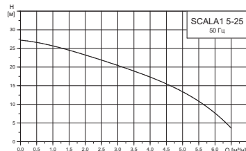
Расходно-напорная характеристика SCALA1 5-25
