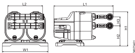
23-сүр. Эки эселенген SCALA1 соркысма орнотмосу
