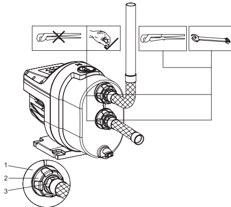
6-сүр. Өткөрмө түтүктөрдү куроо
