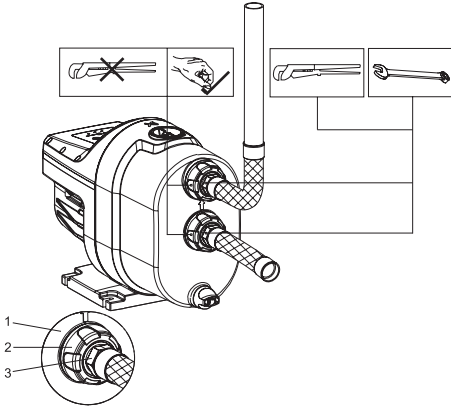
Նկար 6 խողովակաշարերի հավաքակցում
