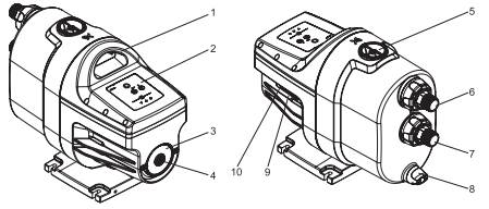
Նկար 1 SCALA1-ի բաղադրիչ մասեր
