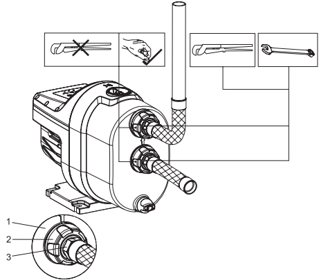
6-сур. Құбыржолдарды құрастыру
