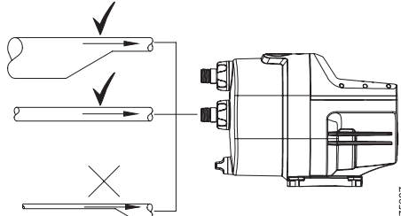
Նկար 7 Շփումից և օդի կուտակումից խուսափելու համար խողովակաշարի խորհուրդ տրվող հավաքակցման ձևը:
