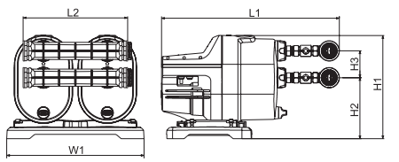
23-сур. SCALA1 қосарланған сорғы қондырғысының өлшемдері
