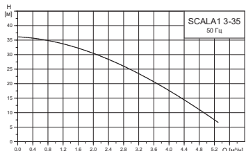
Расходно-напорная характеристика SCALA1 3-35
