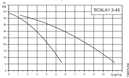
Расходно-напорная характеристика сдвоенной насосной установки SCALA1 3-45
